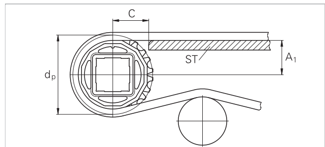
Pignone in un solo pezzo (senza razze)
