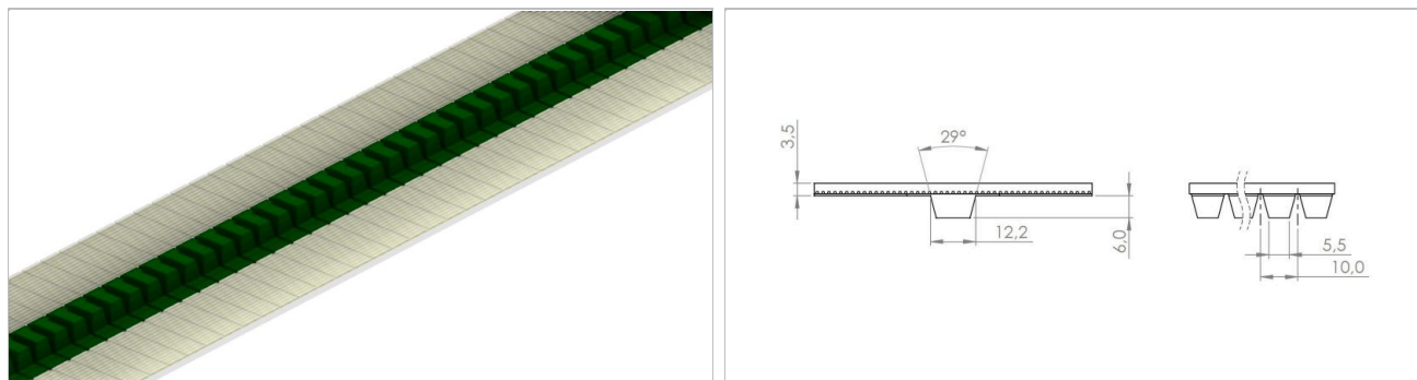
ベルト基本図
