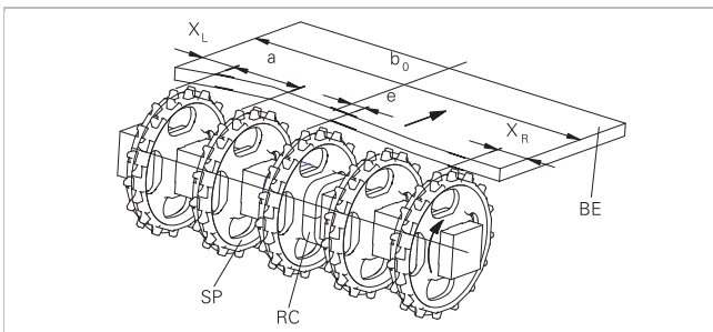
一体型スプロケット (ソリッド) スプロケットの配列
