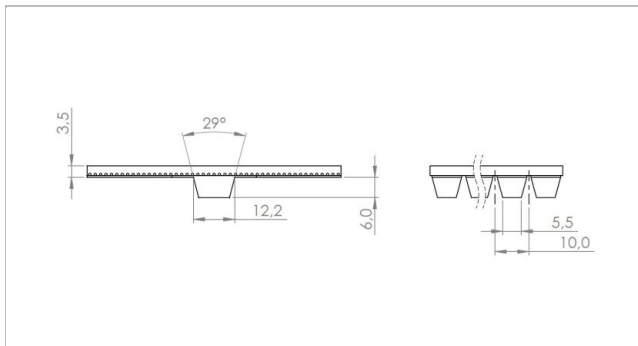
Szkic podstawowego kształtu pasa
