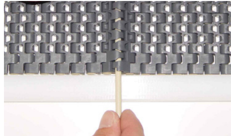
Stab einsetzen. Für ein einfaches Einsetzen des Stabes muss das Ende angefast sein.
