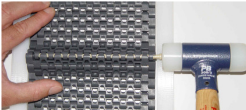
Schlagen Sie den Stabkopf mit einem Hammer hinein
