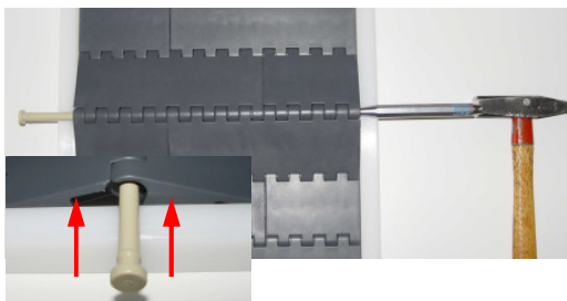
Hebeln Sie den Stabkopf heraus
