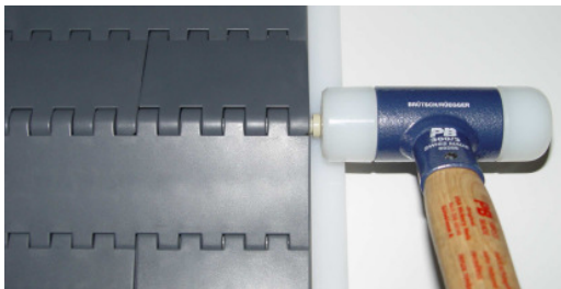
Schlagen Sie den Stabkopf mit einem Hammer hinein
