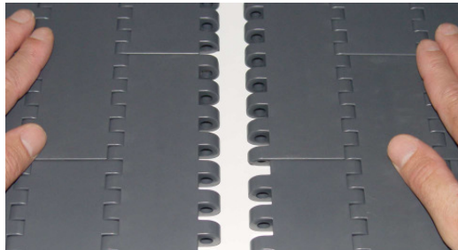
Junte las secciones de banda
