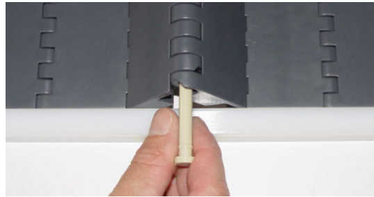
Inserte la varilla. La varilla puede instalarse más fácilmente si el extremo está biselado.
