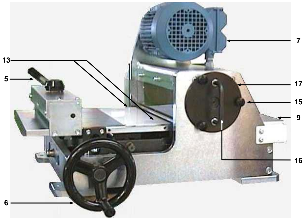
ABBILDUNG 3 – GESAMTANSICHT VON RECHTS
