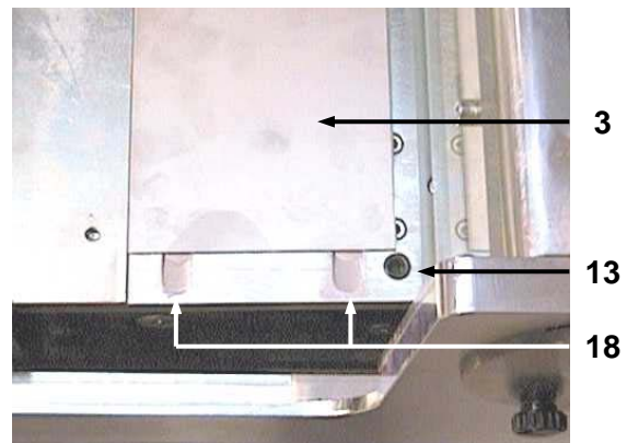
ABBILDUNG 7 – ERSETZEN DER VERSCHLEISSPLATTE
