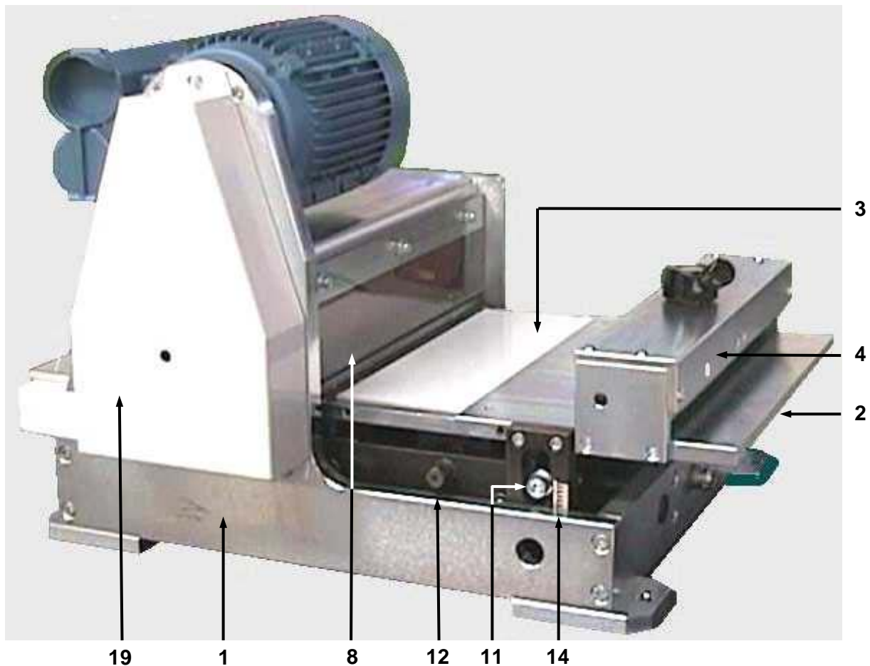
ABBILDUNG 2 – GESAMTANSICHT VON LINKS
