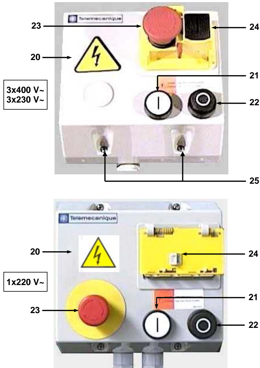
ABBILDUNG 4 – VERSIONEN DES STEUERKASTENS DES AT-305
