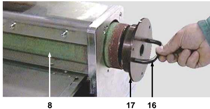
ABBILDUNG 5 – DEMONTAGE DER AUSSCHÄRFWALZE
