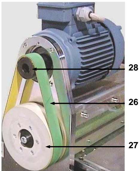
ABBILDUNG 6 – ANTRIEBSRIEMEN
