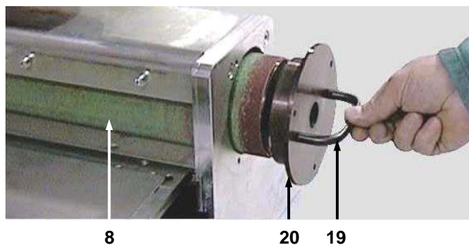
FIGURA 6 – DESMONTAJE DEL RODILLO DE LA BISELADORA
