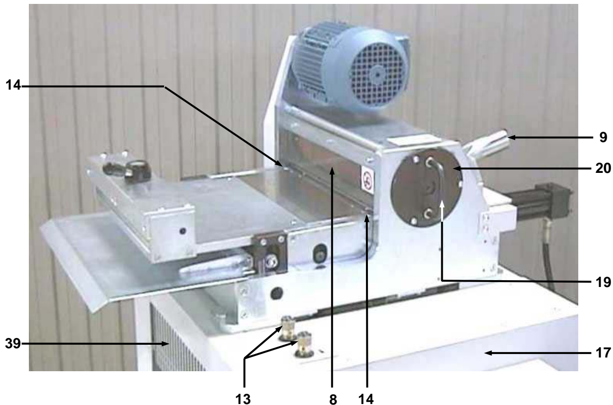
FIGURA 4 – BISELADORA DESDE LA DERECHA
