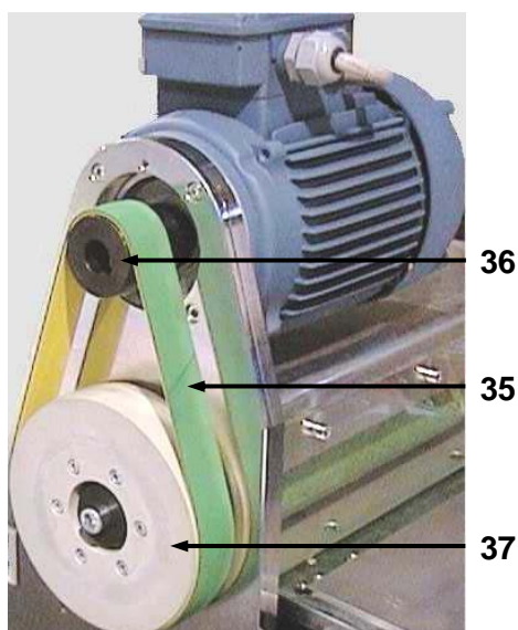
FIGURA 8 – LA CORREA DE TRANSMISIÓN
