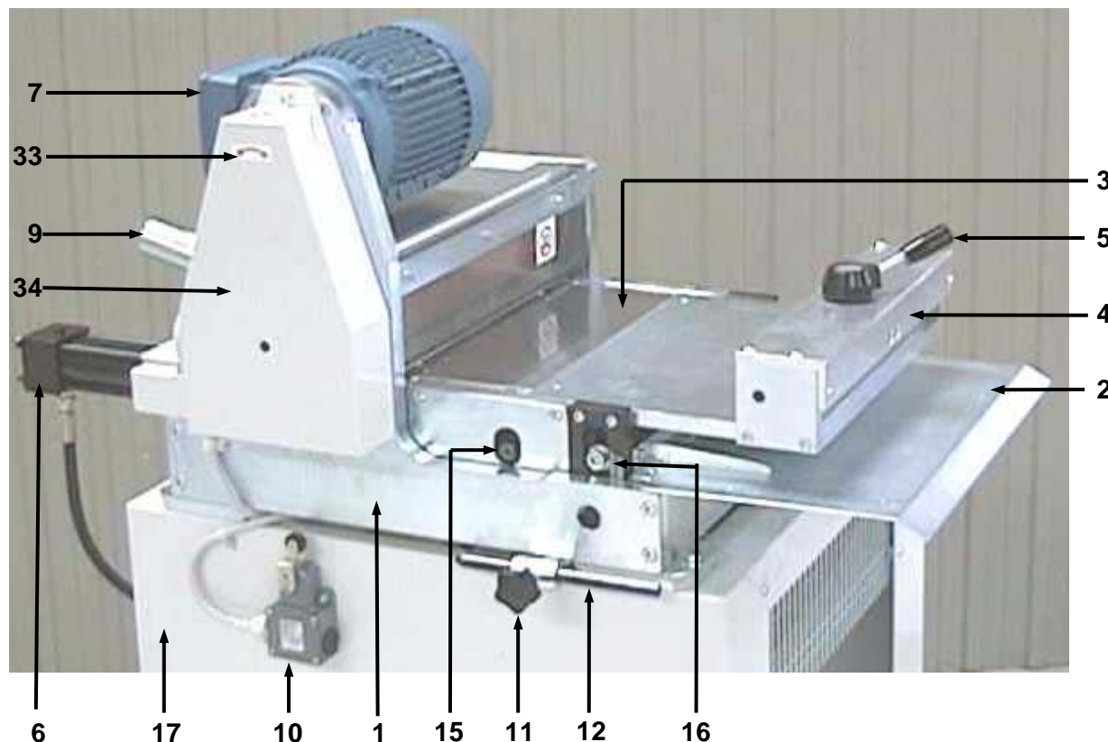
FIGURA 3 – BISELADORA DESDE LA IZQUIERDA
