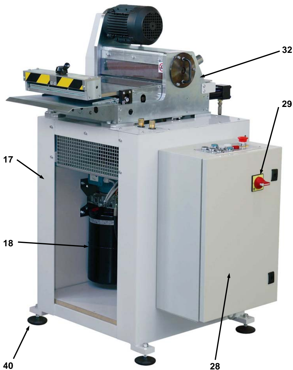
FIGURA 2 – VISTA GENERAL DE LA AT-306
