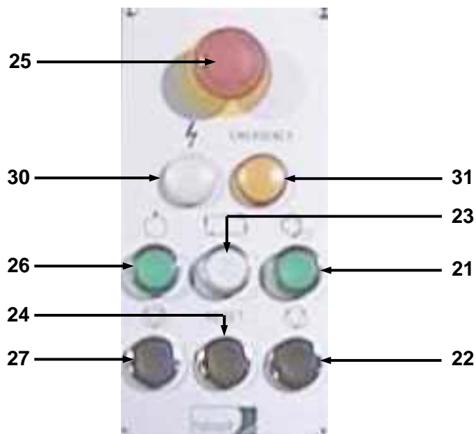
FIGURA 5 – PANEL DE CONTROL DE LA AT-306
