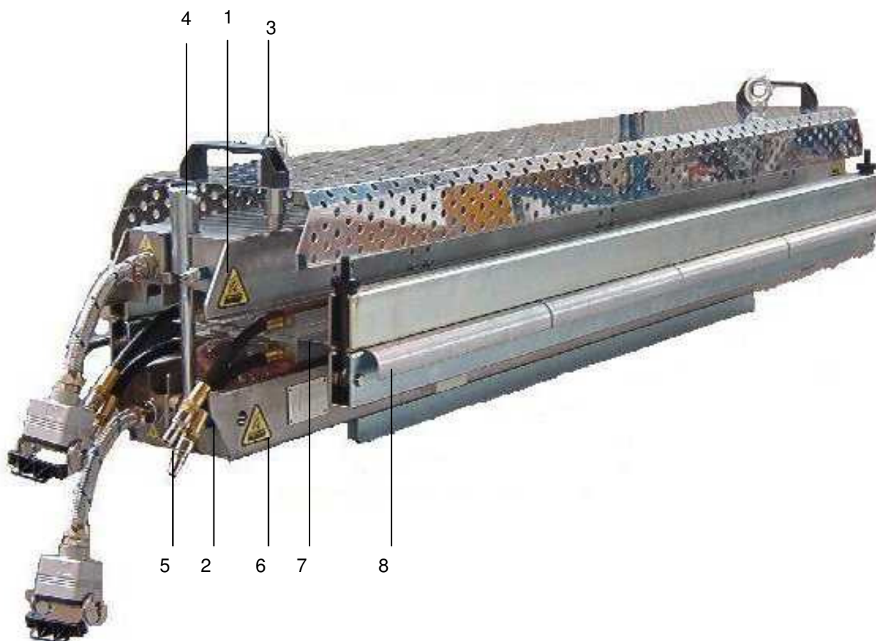
FIGURE 3 - VUE DE LA PRESSE PM-1056/160
