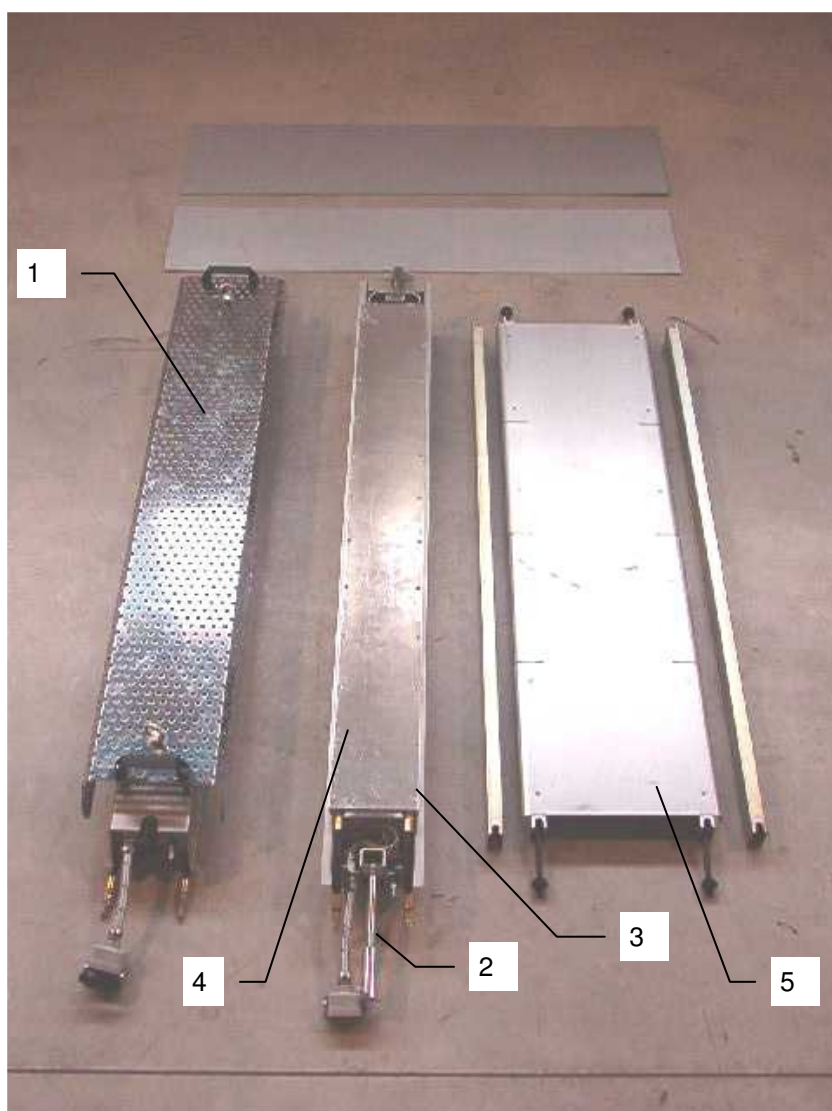
FIGURE 4 - PRINCIPAUX COMPOSANTS DU PM-1056/160
