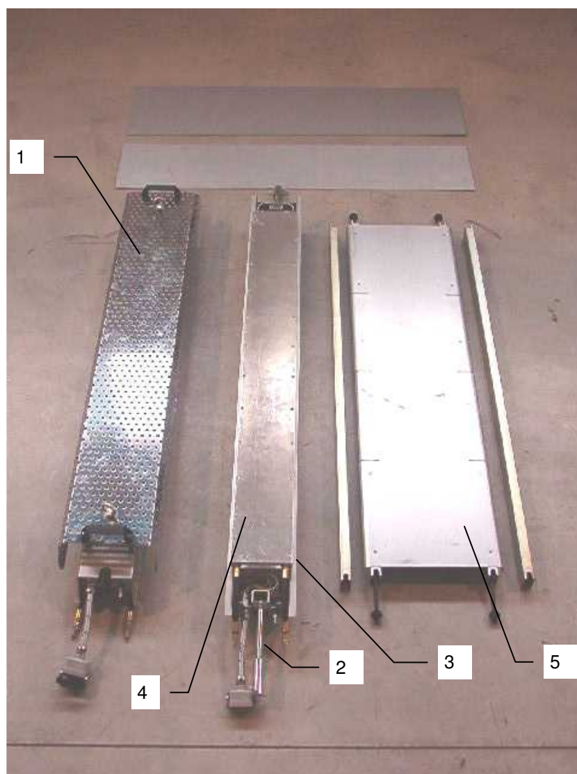
FIGURA 4 - ELEMENTI PRINCIPALI PM 1056/160
