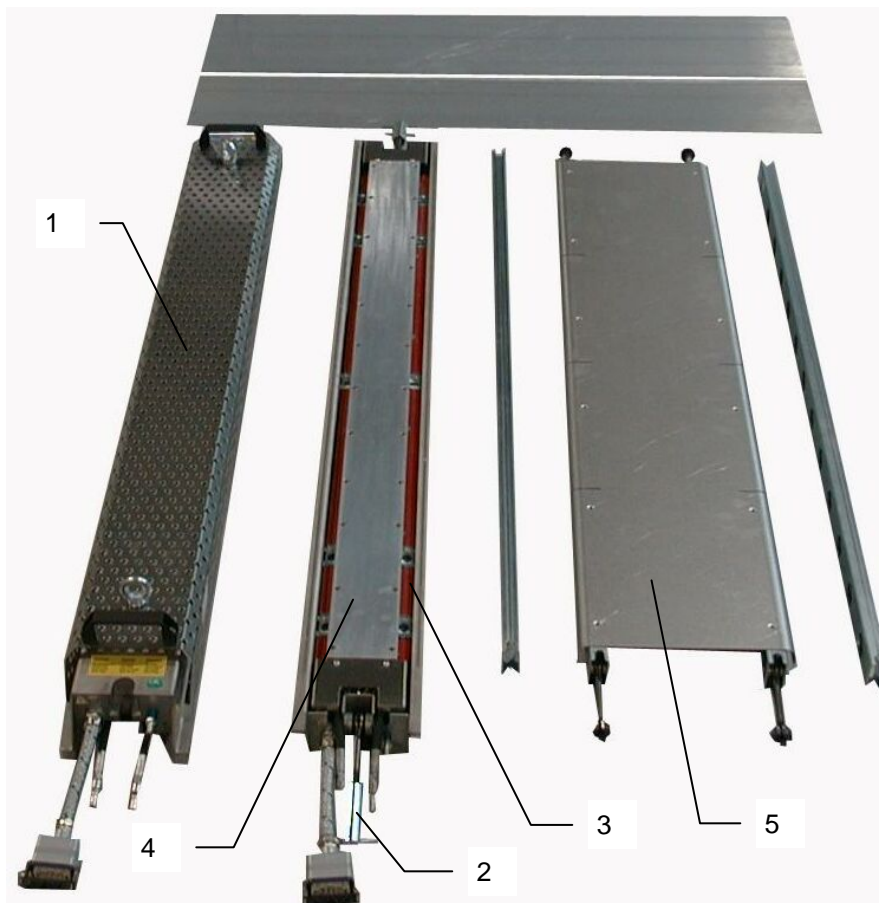
FIGURA 4 - ELEMENTI PRINCIPALI PM-1056
