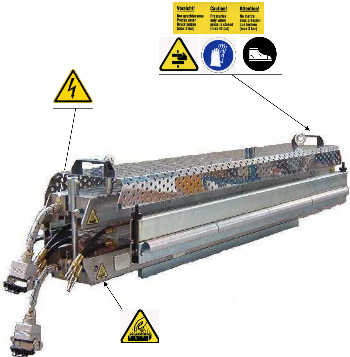
FIGURE 2 - POSITION DES PLAQUES DE SIGNALISATION SUR LA PRESSE
