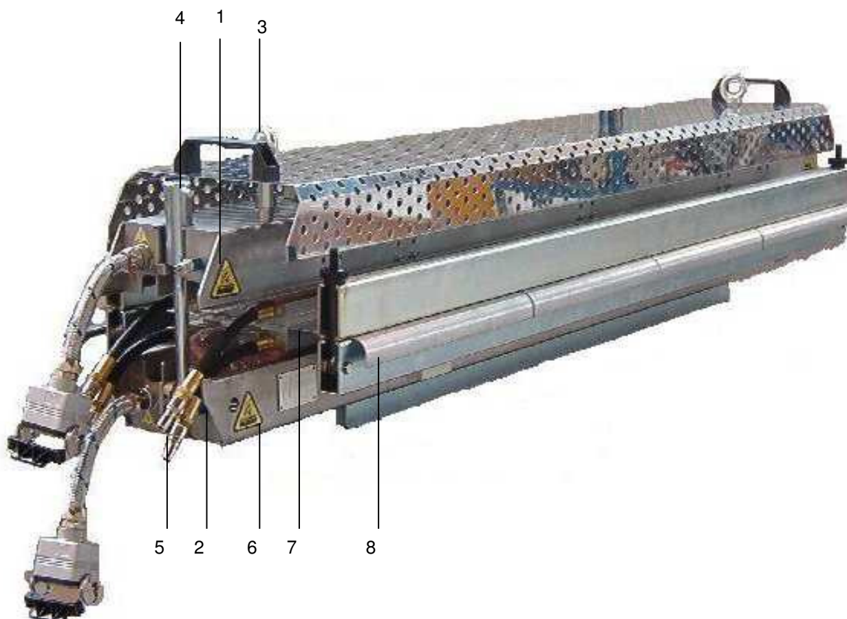
FIGURE 3 - VUE DE LA PRESSE PM-1306/160
