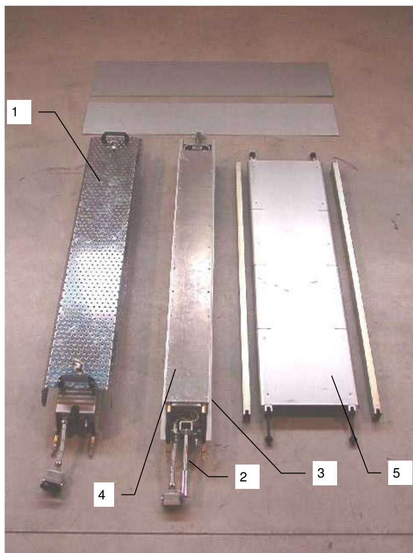
FIGURA 4 - ELEMENTI PRINCIPALI PM 1306/160
