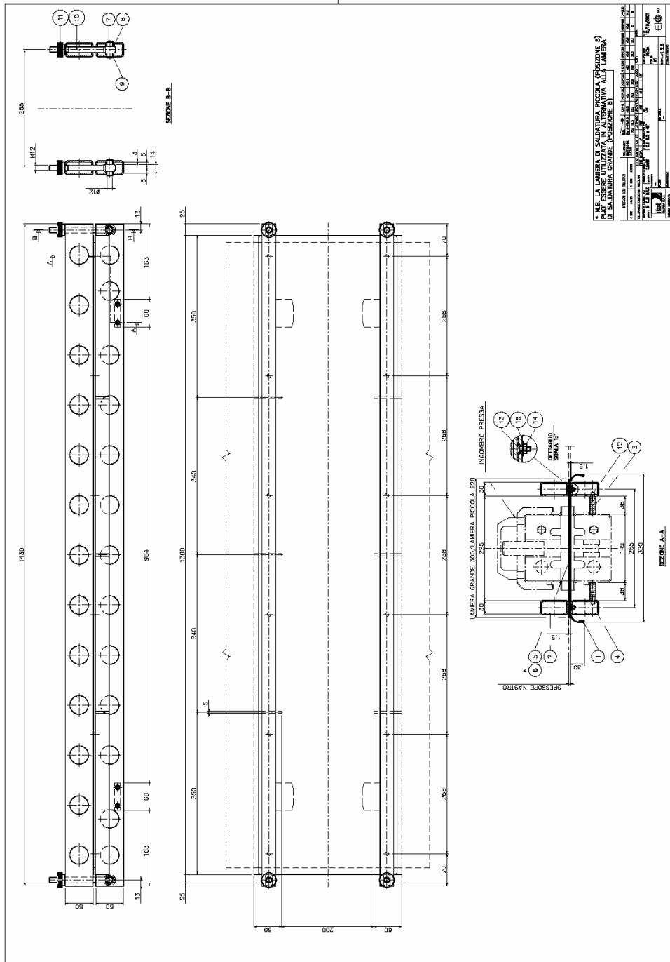
ABBILDUNG 13 – ERSATZTEILE KLEMMVORRICHTUNG
