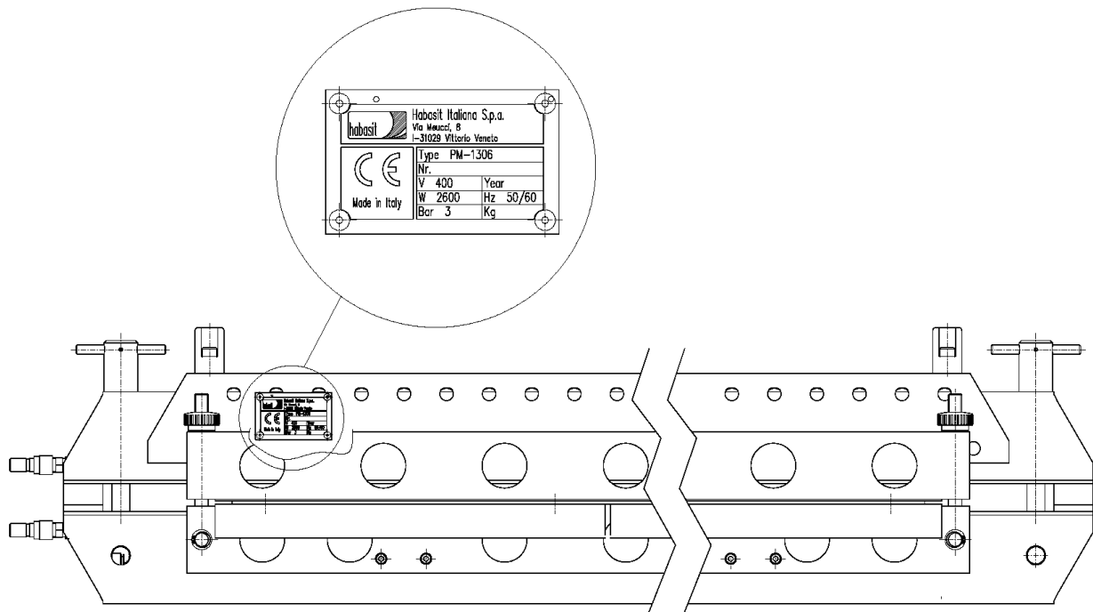
ABBILDUNG 1 – TYPENSCHILD
