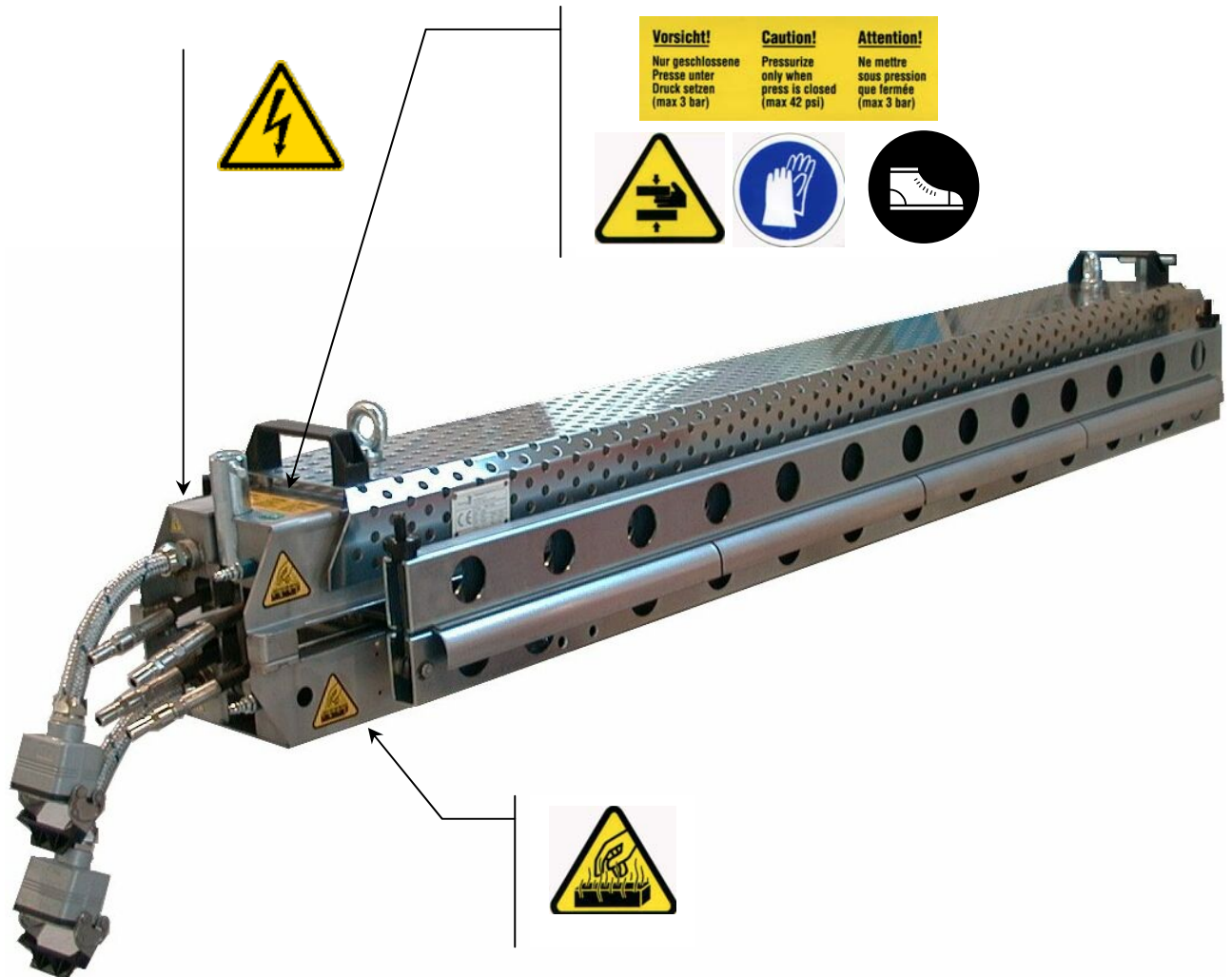
FIGURA 2 - LOCAZIONE SEGNALETICA SULLA PRESSA
