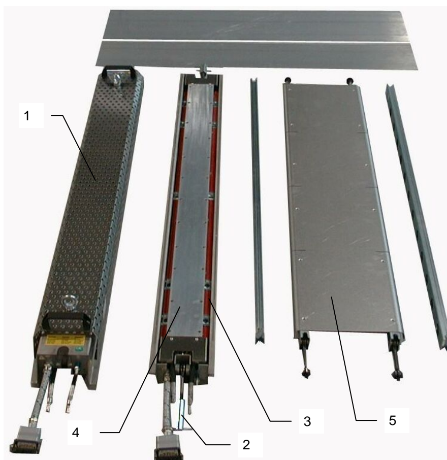
FIGURA 4 - ELEMENTI PRINCIPALI PM 1306
