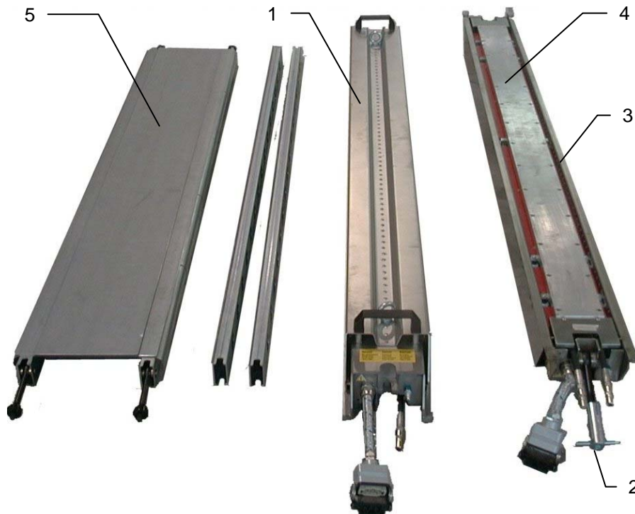
FIGURA 4 - PIEZAS PRINCIPALES DE LA PM-1606
