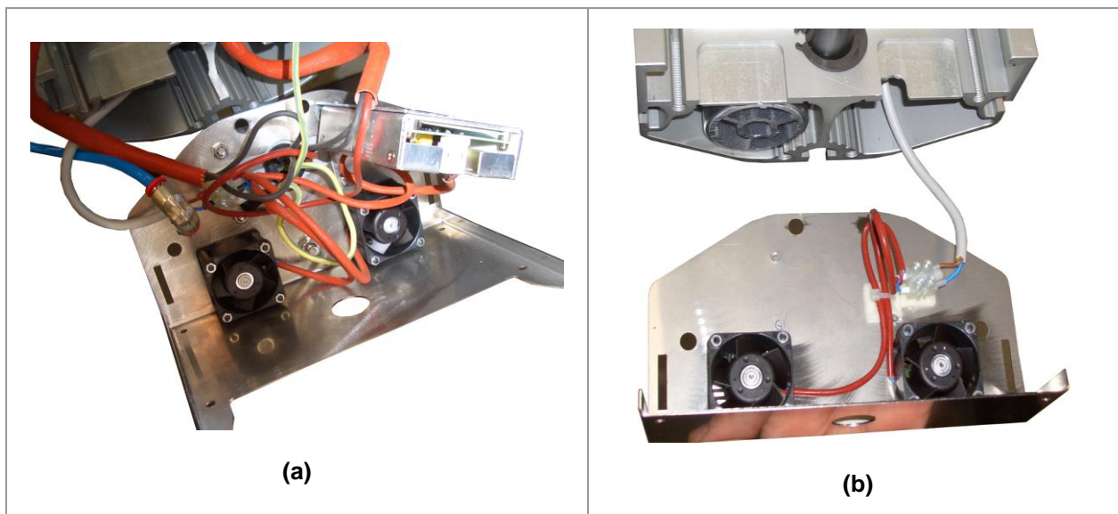
Figure 2 – Branchements internes presse PM-1609/160-B/458, côté connecteurs électriques (a) et côté opposé (b).
