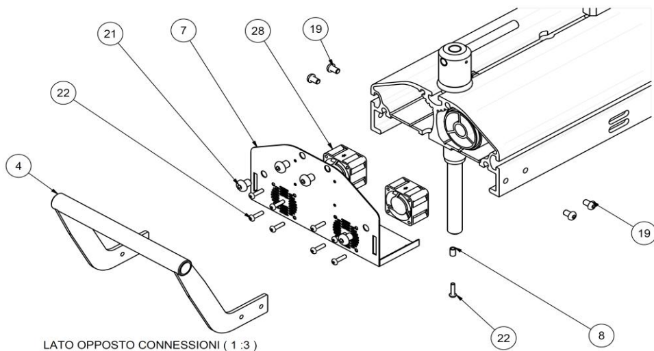
LATO OPPOSTO CONNESSIONI ( 1 : 3 )
