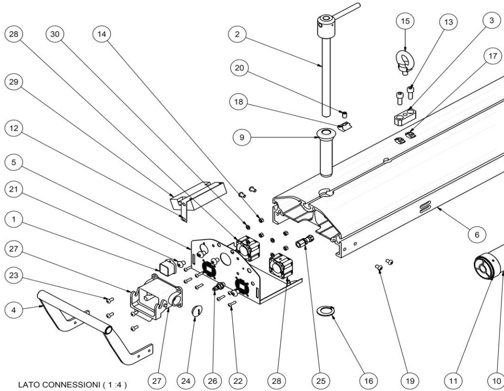
LATO CONNESSIONI ( 1 : 4 )
