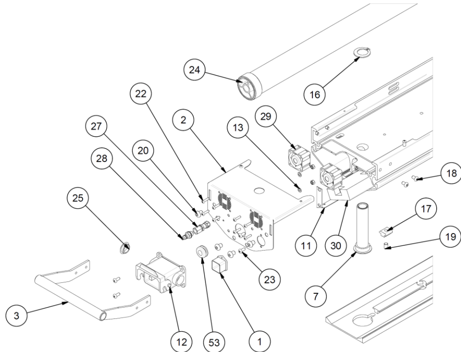
LATO CONNESSIONI ( 1 : 5 )
