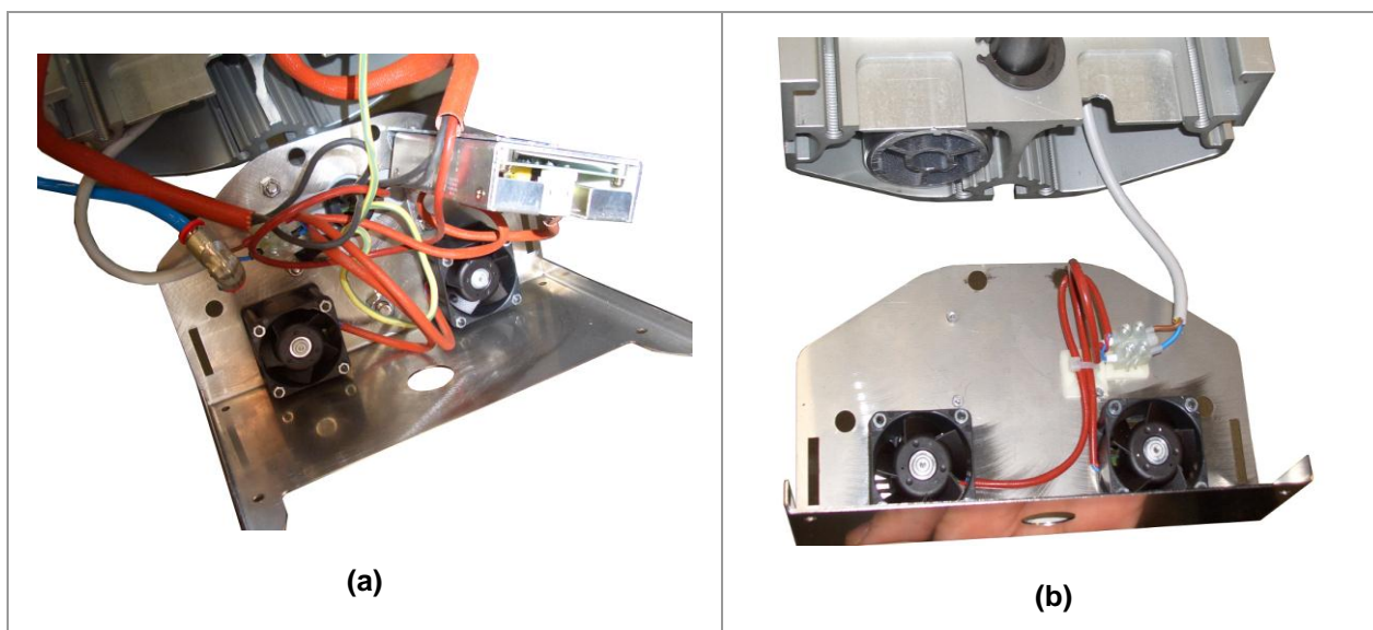
Fig. 2 - Collegamenti interni pressa PM-1609/160-B/45, lato connettori elettrici (a) e lato opposto (b).
