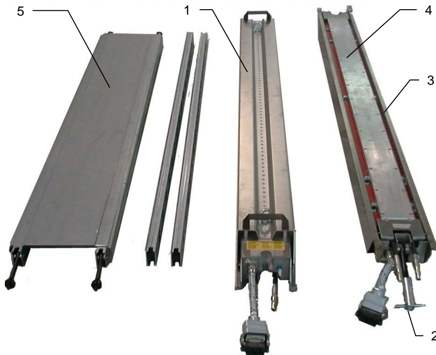
ABBILDUNG 4 – HAUPTBESTANDTEILE DER PM-2006
