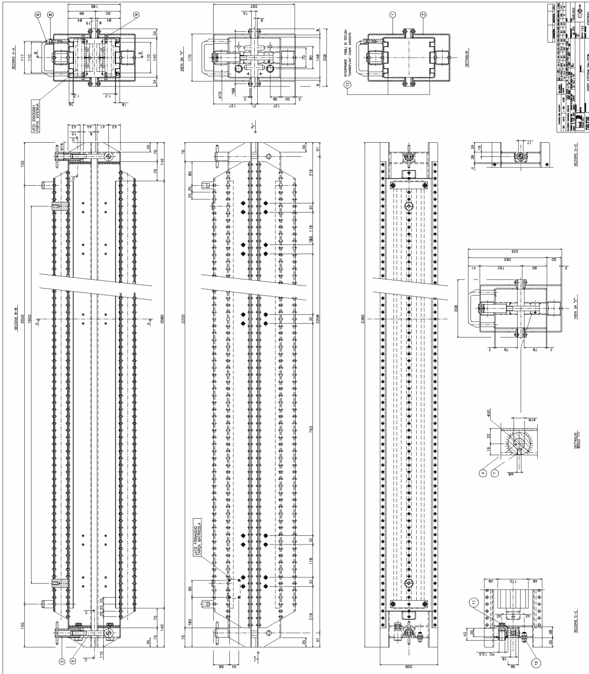
FIGURE 12 - PIÈCES DE RECHANGE EXTERNES
