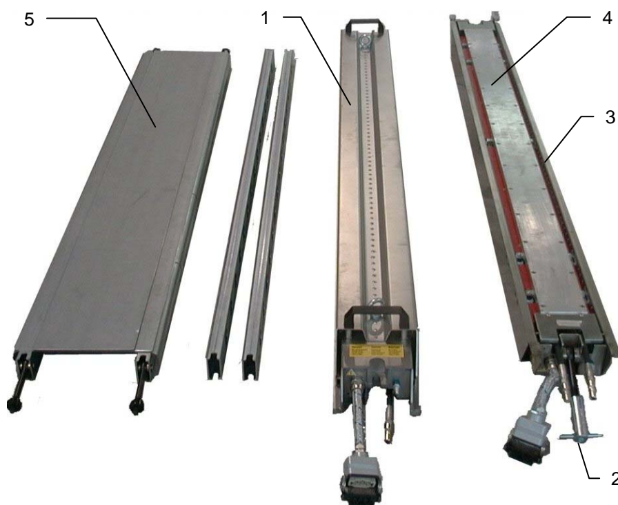
FIGURE 4 - PRINCIPAUX COMPOSANTS DU PM-2006
