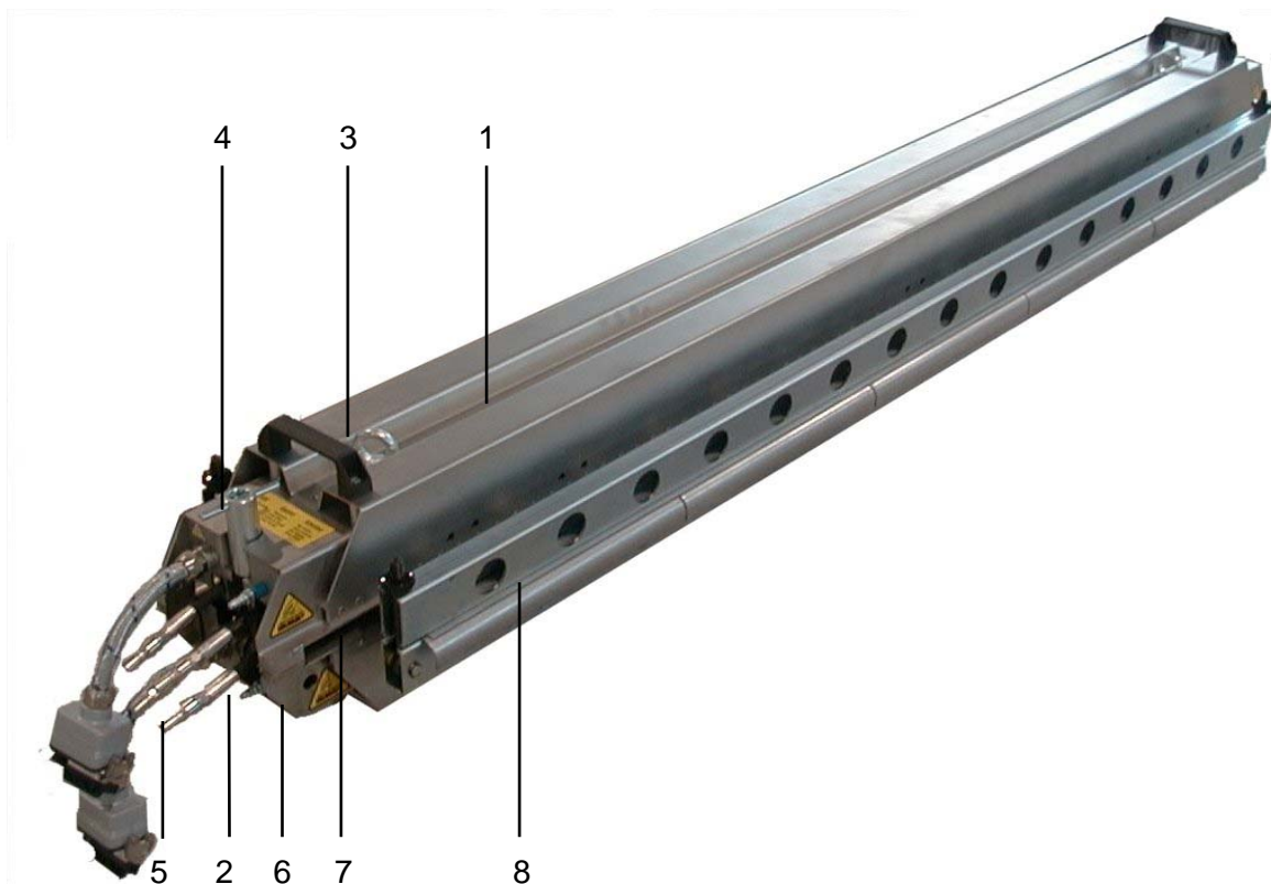
FIGURE 3 - VUE DE LA PRESSE PM-2006
