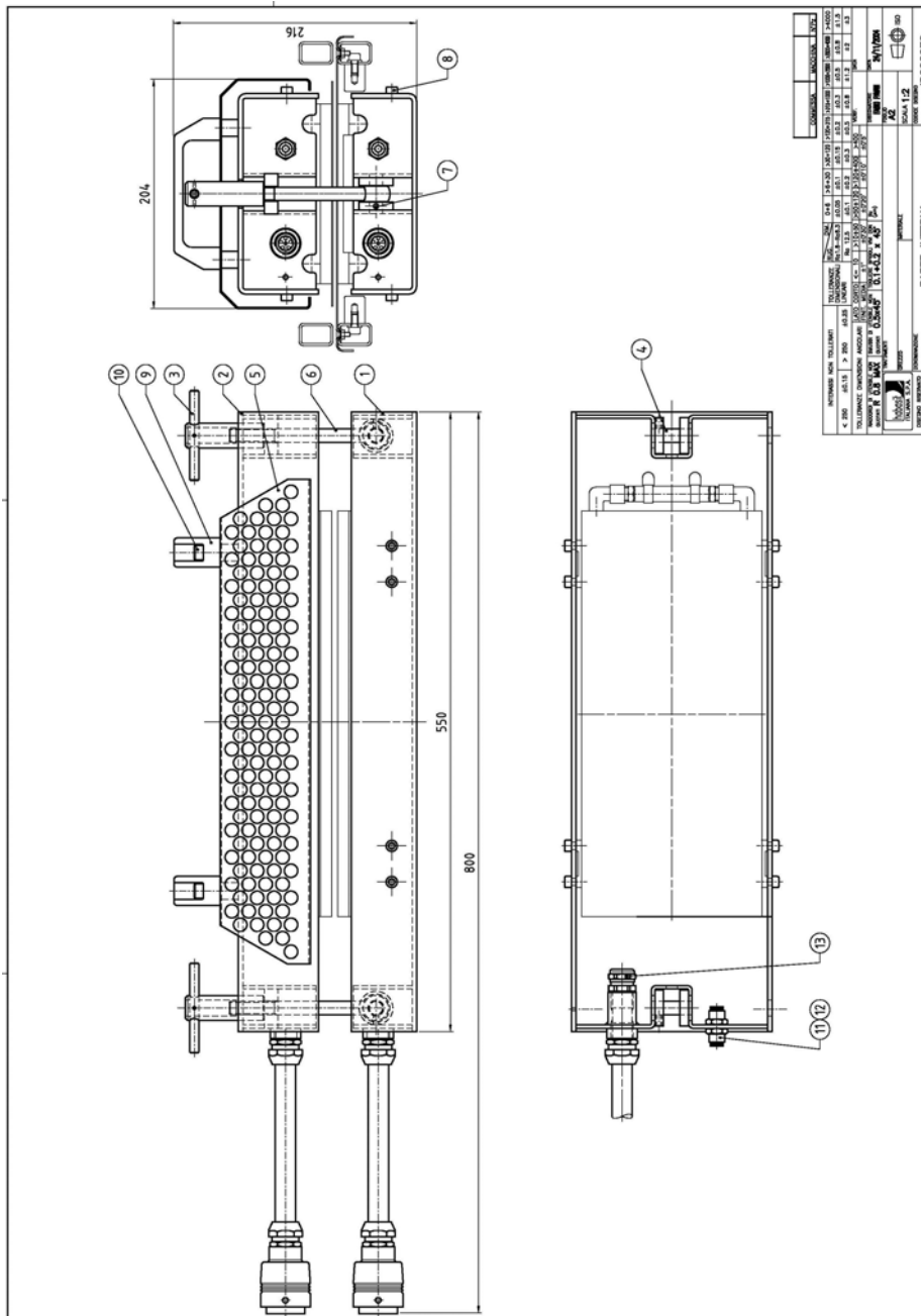
ABBILDUNG 11 – ERSATZTEILE AUSSEN
