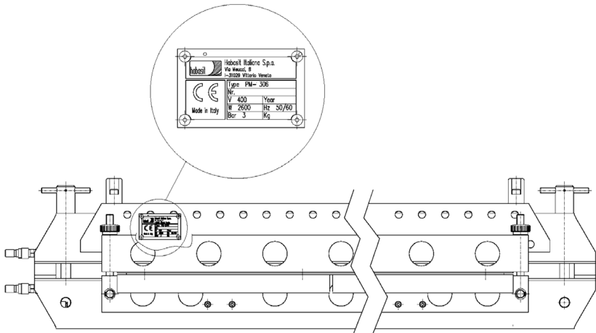
ABBILDUNG 1 – TYPENSCHILD
