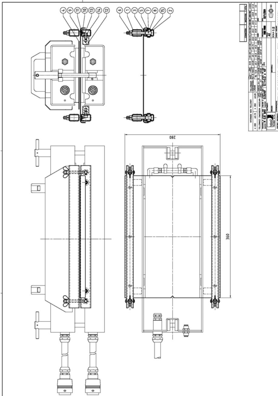
ABBILDUNG 12 – ERSATZTEILE KLEMMVORRICHTUNG
