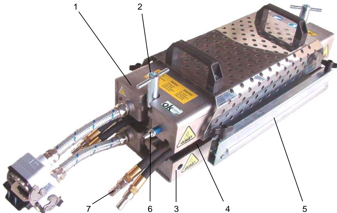
ABBILDUNG 3 – DARSTELLUNG DER PM-306/160
