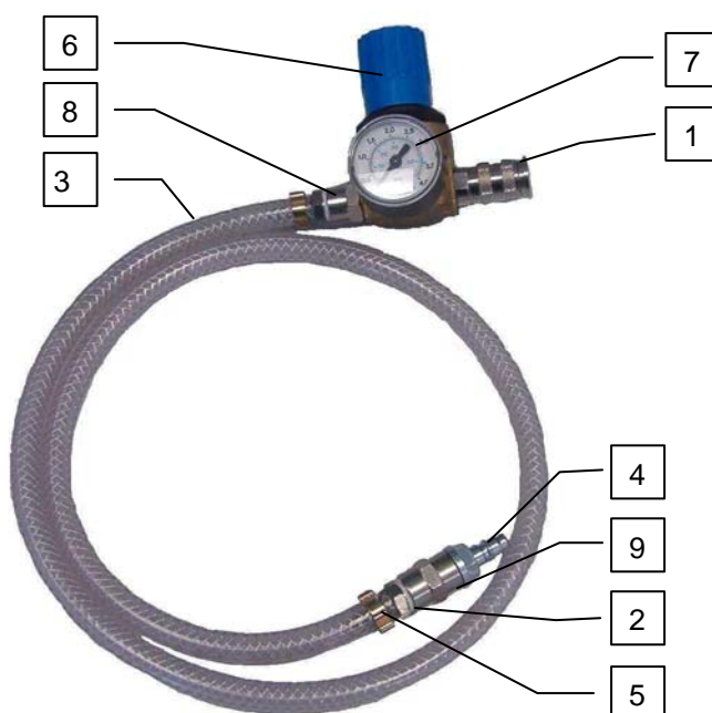
ABBILDUNG 13 – ERSATZTEILE FÜR DRUCKLUFTANSCHLUSS
