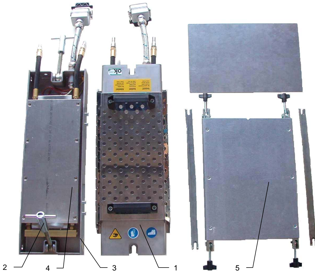
ABBILDUNG 4 – HAUPTBESTANDTEILE DER PM-306/160
