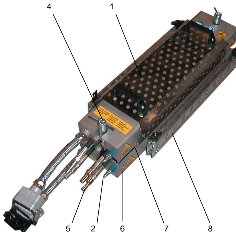
ABBILDUNG 3 – DARSTELLUNG DER PM-306
