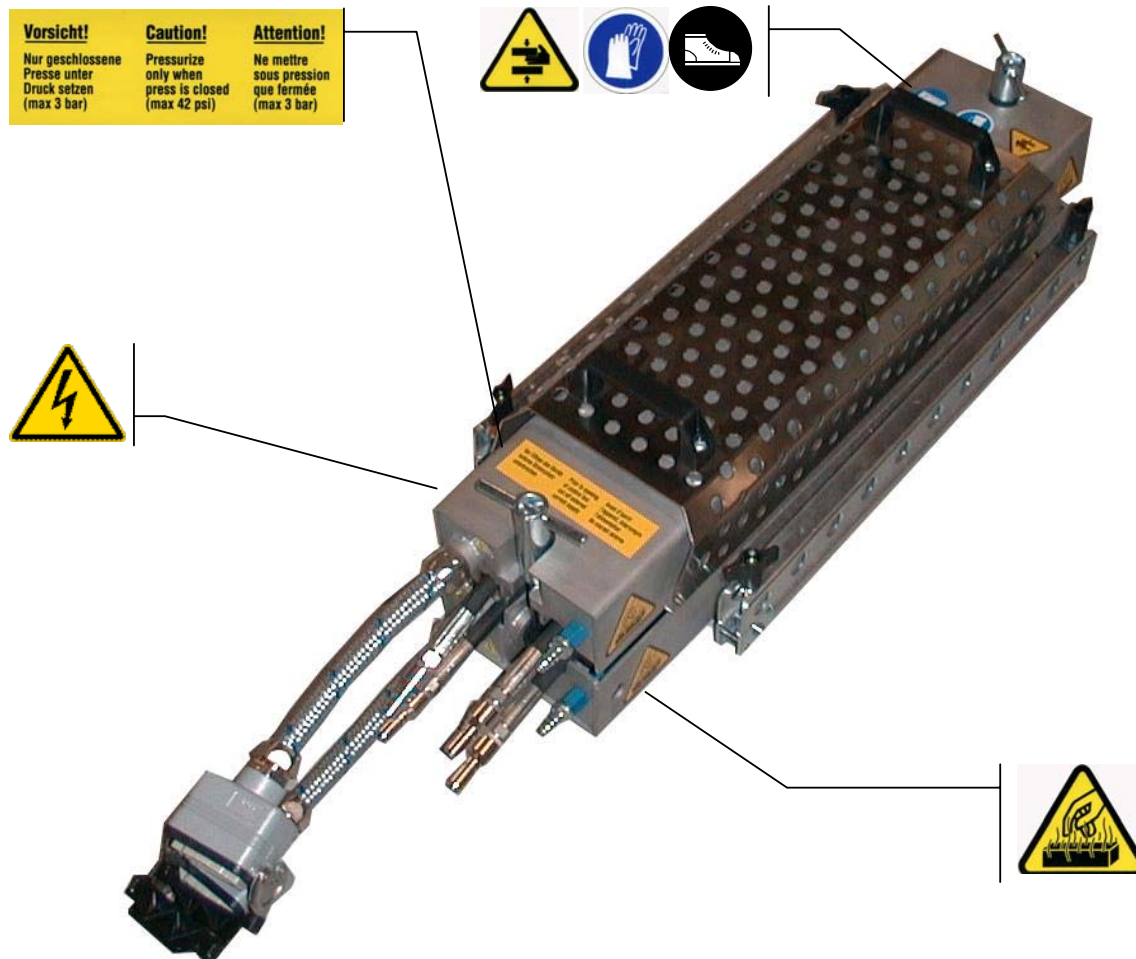
ABBILDUNG 2 – POSITION VON SCHILDERN AN DER PRESSE
