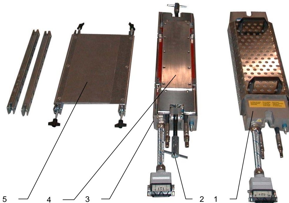
ABBILDUNG 4 – HAUPTBESTANDTEILE DER PM-306
