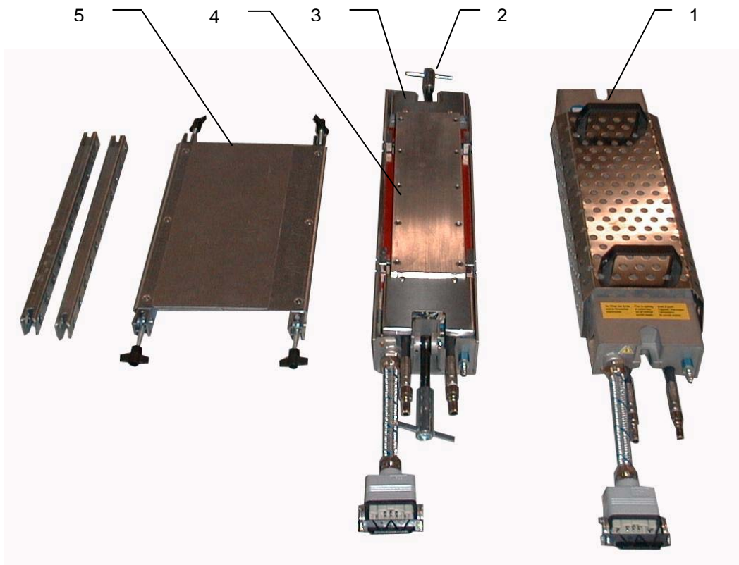
FIGURA 4 - ELEMENTI PRINCIPALI PM-306
