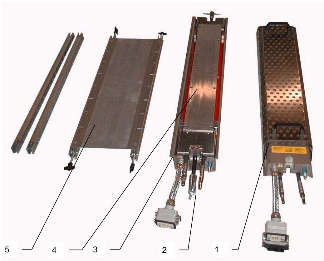
FIGURA 4 - PIEZAS PRINCIPALES DE LA PM-606
