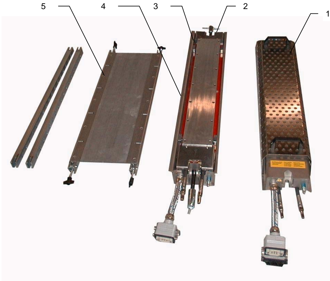
FIGURA 4 - ELEMENTI PRINCIPALI PM-606
