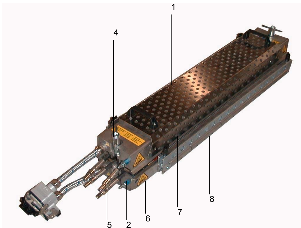
FIGURA 3 - VISTA COMPLESSIVA PM-606
