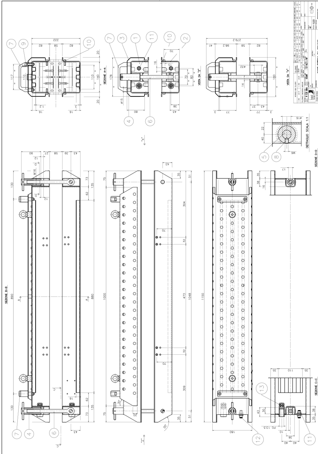
ABBILDUNG 12 – ERSATZTEILE AUSSEN
