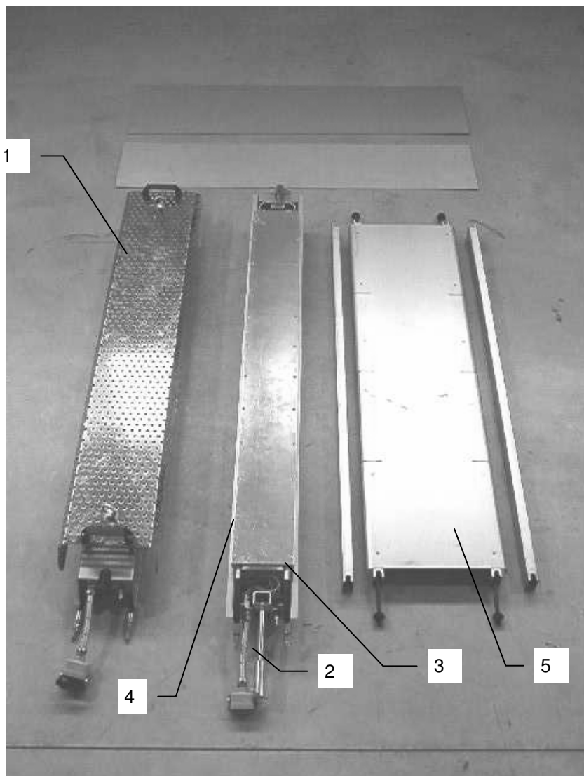
ABBILDUNG 4 – HAUPTBESTANDTEILE DER PM-806/160
