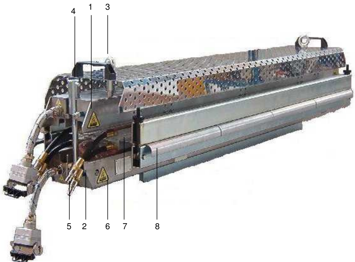
ABBILDUNG 3 – DARSTELLUNG DER PM-806/160
