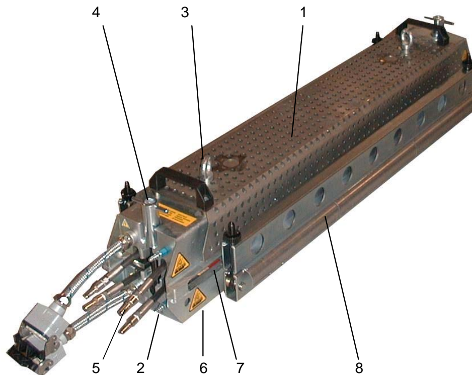
ABBILDUNG 3 – DARSTELLUNG DER PM-806
