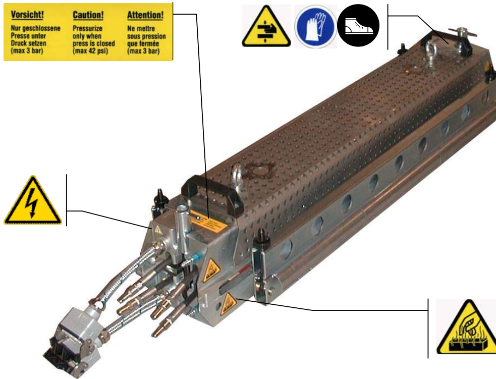
ABBILDUNG 2 – POSITION VON SCHILDERN AN DER PRESSE
