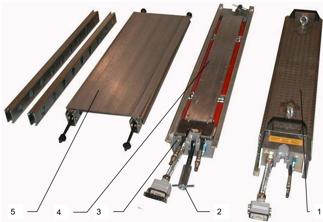
ABBILDUNG 4 – HAUPTBESTANDTEILE DER PM-806
