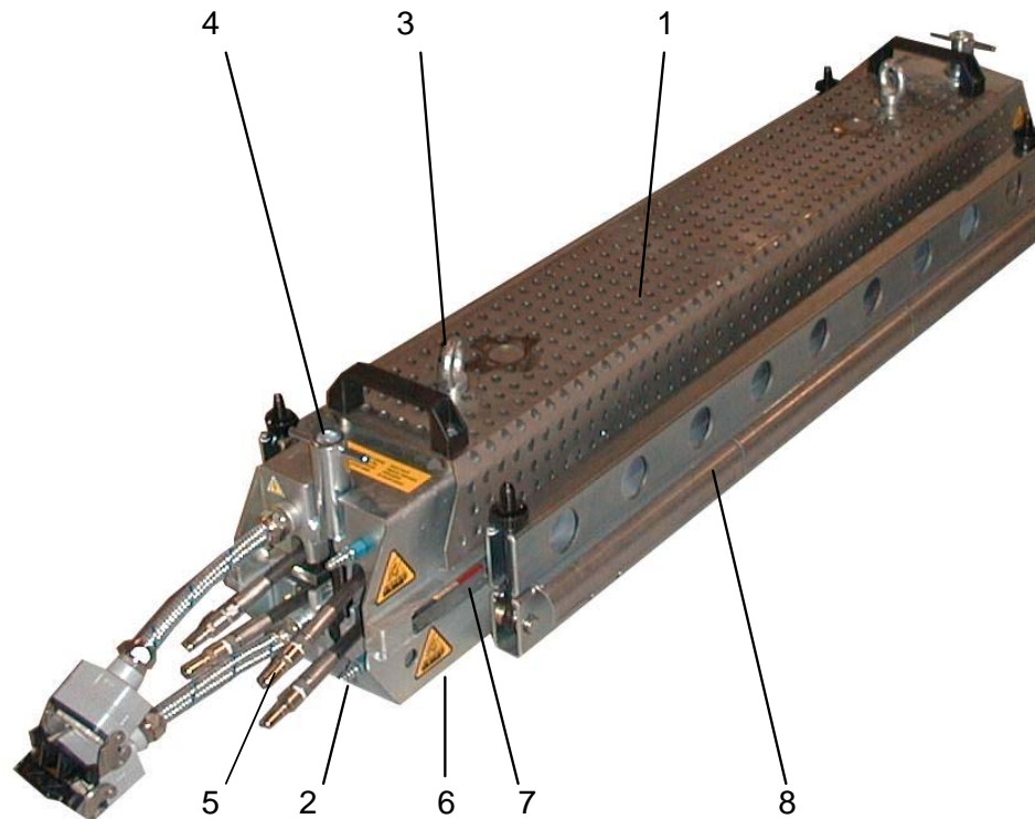
FIGURA 3 - VISTA DE LA PM-806
