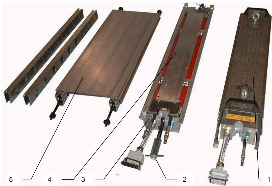
FIGURA 4 - PIEZAS PRINCIPALES DE LA PM-806
