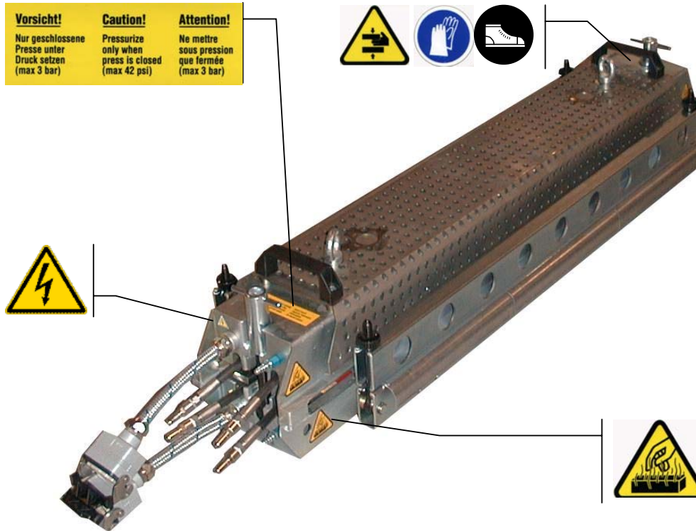
FIGURA 2 - POSICIÓN DE LAS SEÑALES EN LA PRENSA
