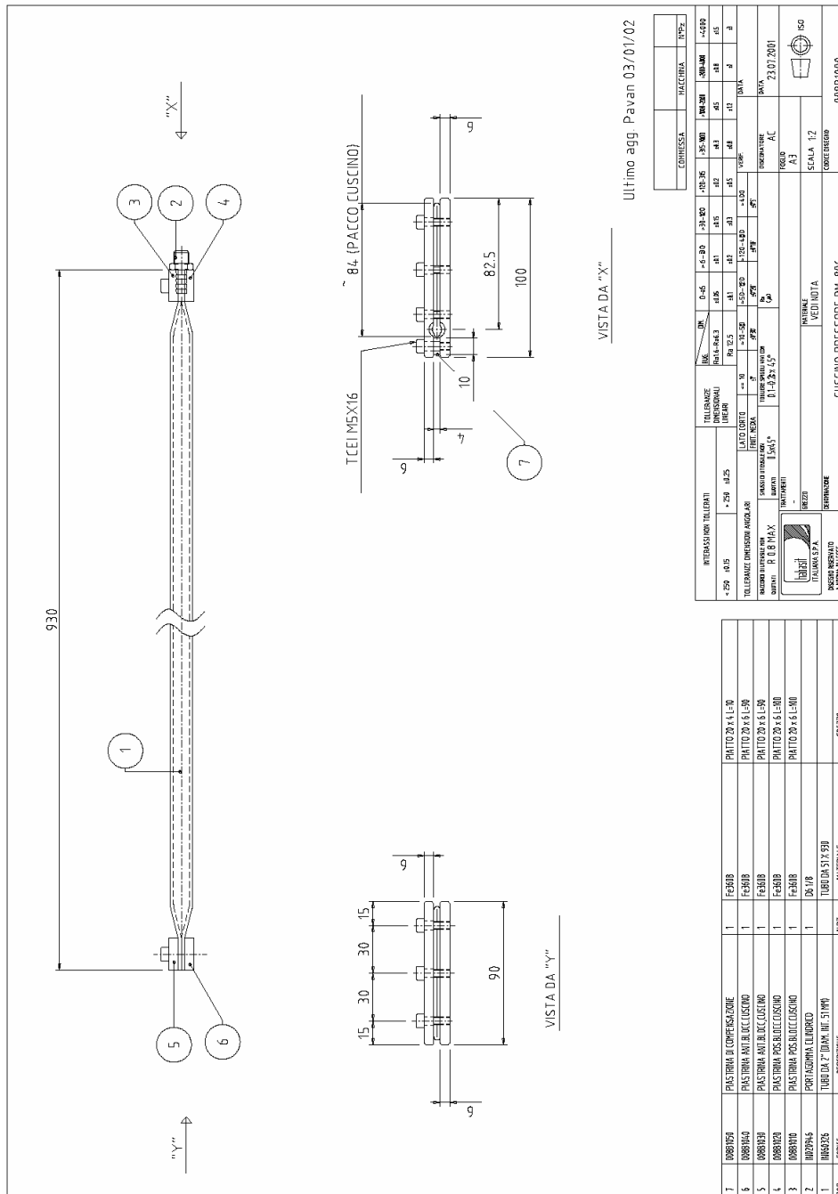
FIGURA 11 - PIEZAS DE REPUESTO DEL COJÍN A PRESIÓN
