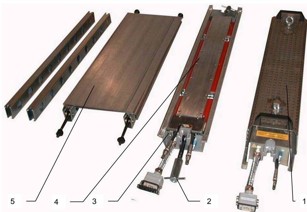
FIGURE 4 - PRINCIPAUX COMPOSANTS DU PM-806
