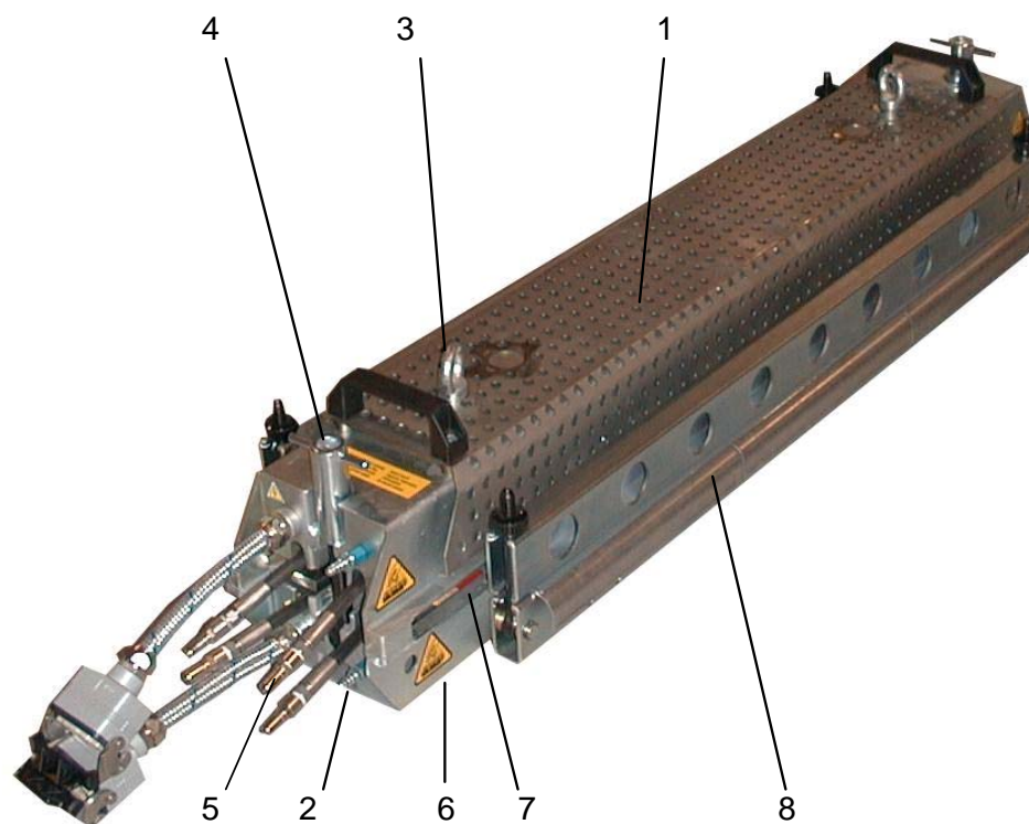
FIGURE 3 - VUE DE LA PRESSE PM-806
