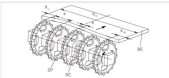
一体型スプロケット ("窓あき") スプロケットの配列
