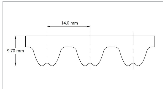
Schets van tandprofiel
