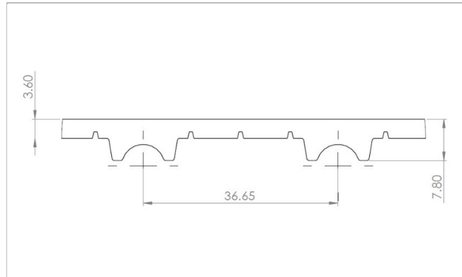
基本形状草图
